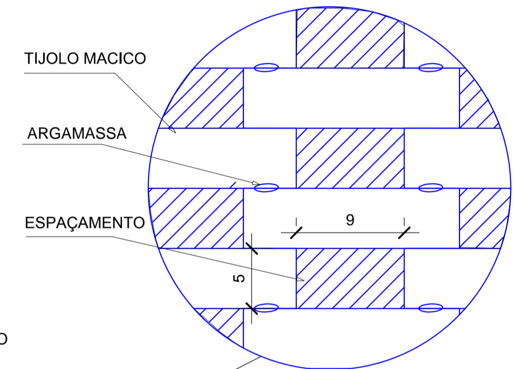
DETALHE DA ALVENARIA VAZADA
