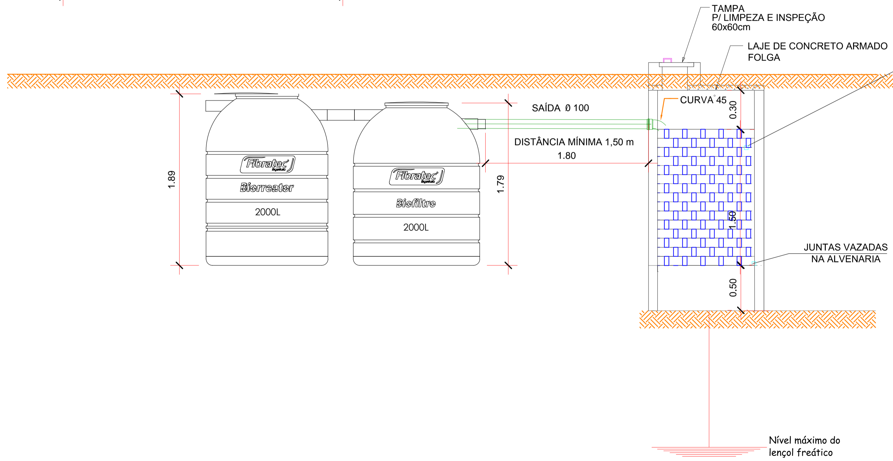
DETALHE DA ALVENARIA VAZADA
