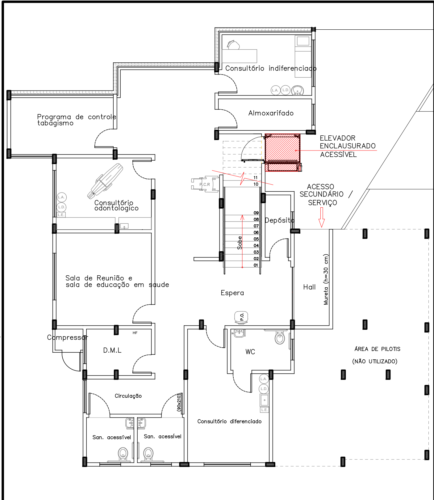
PLANTA BAIXA - INFERIOR ESCALA 1:100
