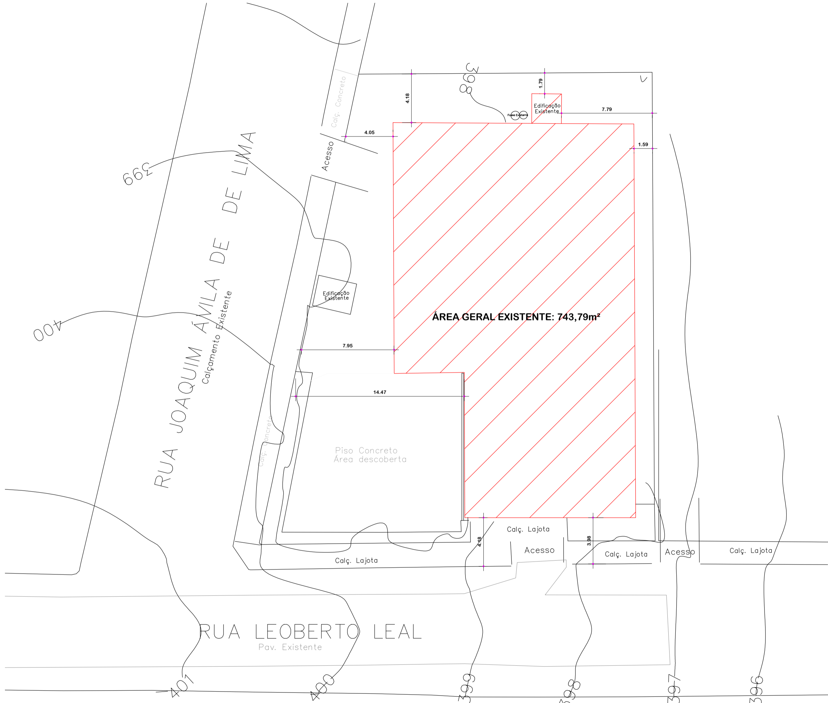
PLANTA DE SITUAÇÃO/LOCAÇÃO ESC 1/200
