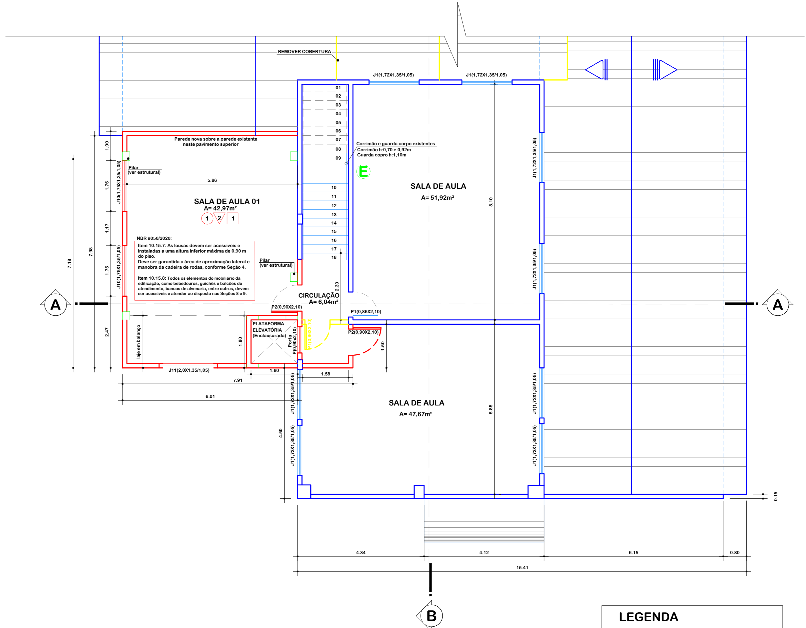
PLANTA BAIXA - PVTO SUPERIOR ÁREA PVTO SUPERIOR EXISTENTE: 121,79m² ÁREA PVTO SUPERIOR AMPLIAÇÃO: 47,96m² ÁREA PVTO SUPERIOR TOTAL: 169,75m² ÁREA TOTAL DA OBRA: 874,52m² ESC.: 1:75
