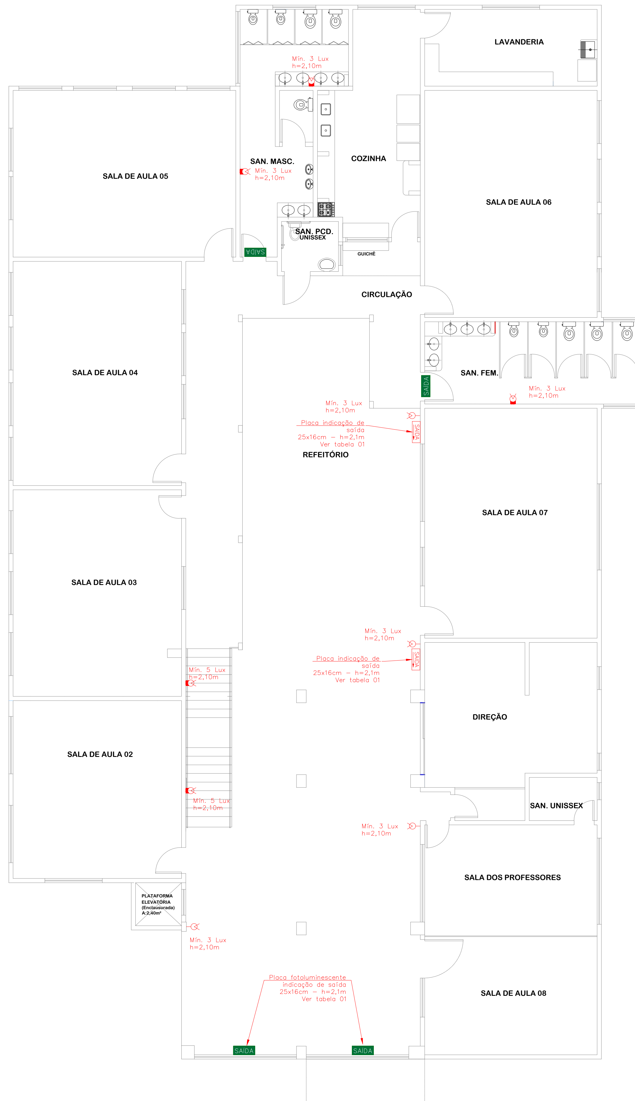
PLANTA BAIXA - PVTO TÉRREO ESC.: 1:75
