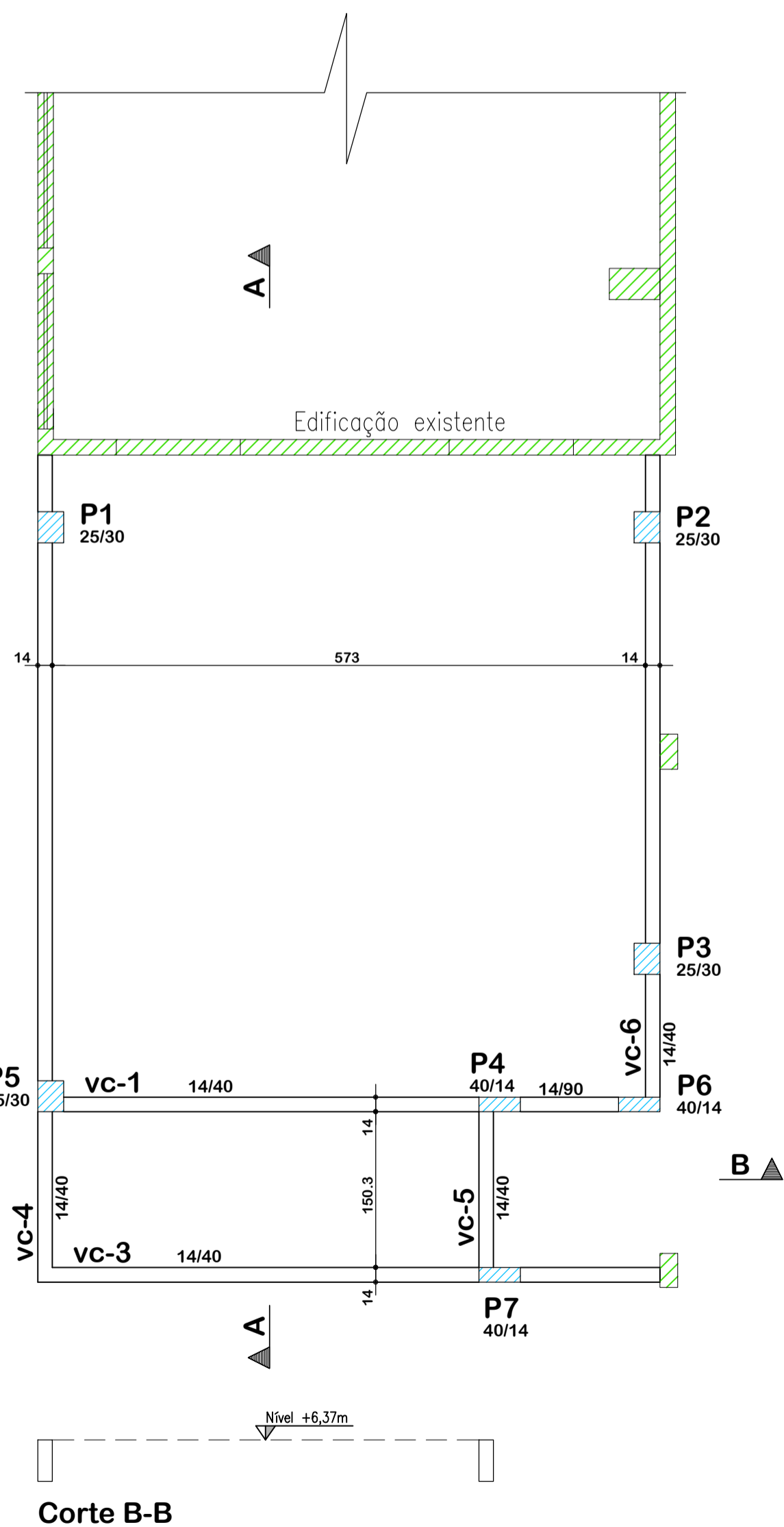
Planta de formas: Cobertura Escala: 1:50
